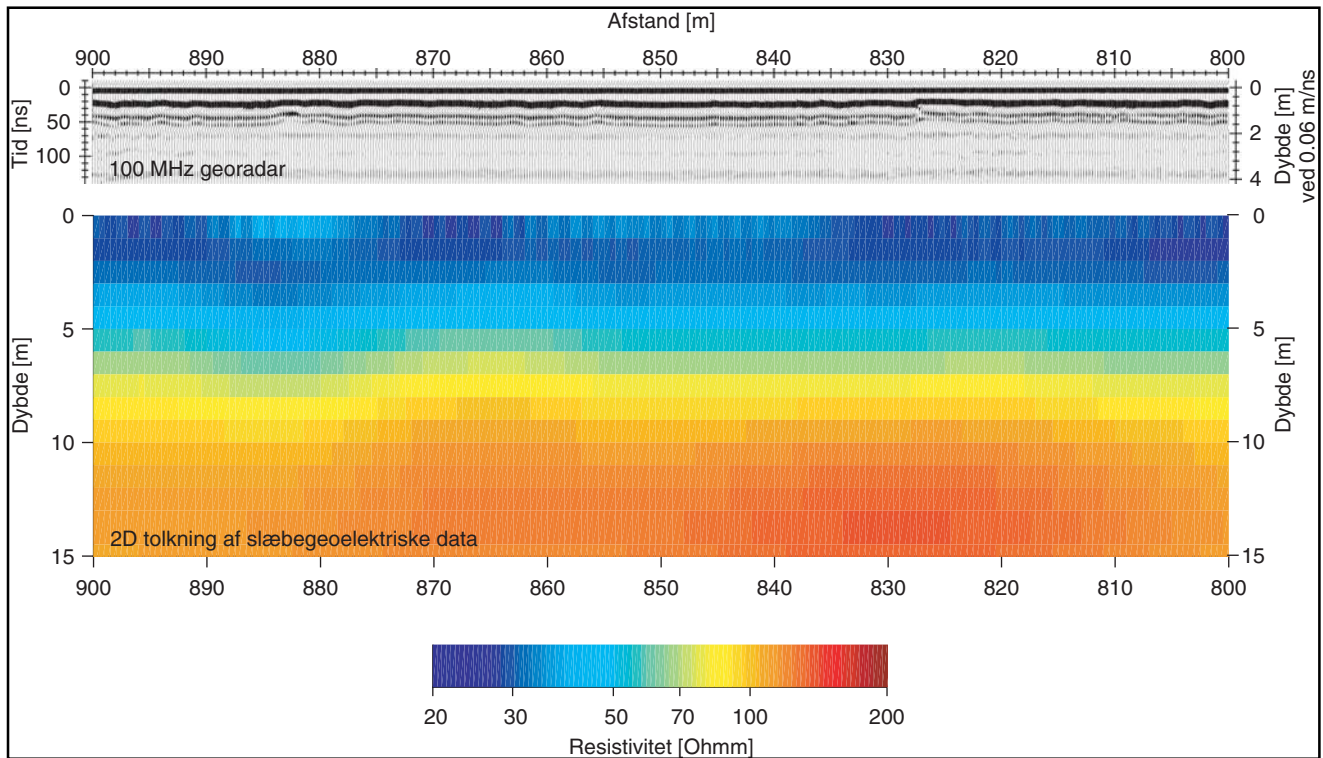
Et 100 m udsnit af georadarprofil og slæbegeoelektrisk profil vest for Rødvig på Stevns. Profilerne er placeret i et område, hvor otte til ti meter moræneler overligger Danienkalk. Der er målt lave resistiviteter med slæbegeoelektrik og meget ringe indtrængningsdybde med georadar. Georadardataene er indsamlet med et 100 MHz georadarsystem. De viste data er forstærket (gainet) ved brug af en rutine, der bevarer de relative amplitudestyrkeforhold, og migrerer med konstant hastighed på 0.06 m/ns. En hastighed på 0.06 m/ns er også anvendt til dybdekonverteringen. Det slæbegeoelektriske profil viser et udsnit af en 2D-model, som er resultatet af en tolkning af de slæbegeoelektriske data udført med 2D inversionsprogrammet DCIP2D. (Grafik: Forfatterne)
