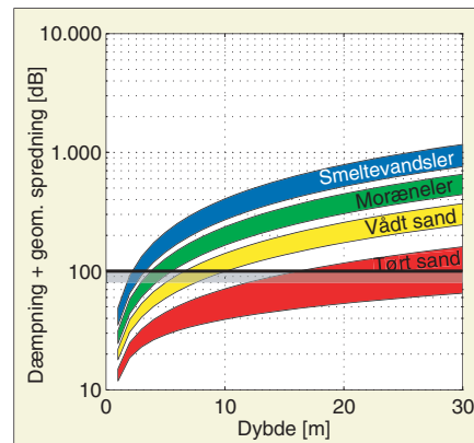
Samlet elektrisk dæmpning og geometrisk spredning for fire jordtype-scenarier (summen af kurverne i de to figurer til venstre). Kurverne viser, hvor meget signalet reduceres på vejen ned mod en reflektor. Den fede sorte streg markerer en signalreduktion på 100 dB, og den grå skyggezone angiver niveauet ned til 80 dB. 80 dB svarer til et realistisk mål for det halve af en georadars "system performance". Figuren viser kun de elementer af signalreduktionen, der kan beregnes via simple relationer. Spredning som følge af finskala heterogenitet er ikke medtaget i beregningerne. Derfor er den dybde, hvor signalet ligger i skyggezone, et optimistisk bud på en indtrængningsdybde. (Grafik: Forfatterne)
