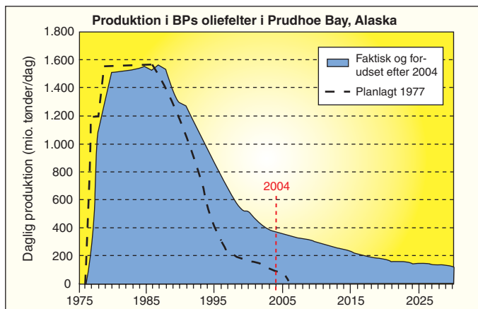
Produktion i BPs olie-felter i Prudhoe Bay, Alaska. Ved en kraftig og dyr indsats med nye udvindings teknikker er det lykkedes at forøge udvindingsgraden af den olie, der findes i felterne, fra 45 % til 60 %, og således at bremse produktionsfaldet. Men sådanne dyre udvindings teknikker bringes først i anvendelse, når olien i længere tid "kommer op af sig selv", dvs. når produktionen er toppet. (Grafik: UVH modificeret efter Francis Harper, tidligere direktør i BP)
