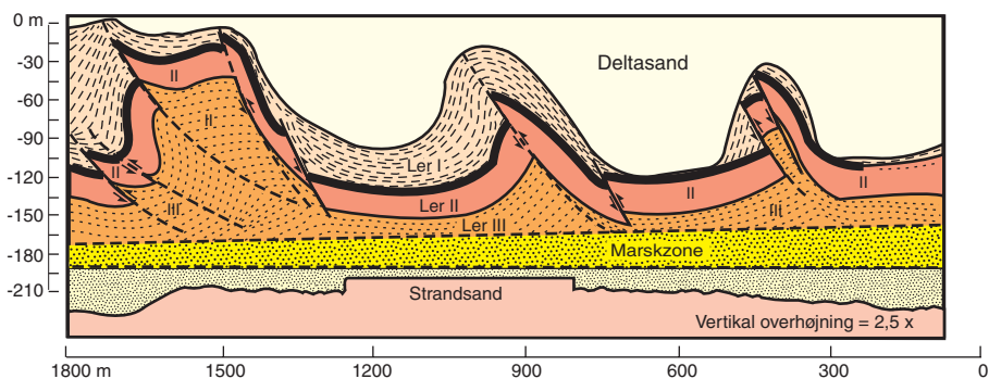
Slumpfolder og overskydninger i sedimenter i Mississippideltaet. Af uforklarlige grunde har de konventionelle kvartærgeologer ikke diskuteret, hvorvidt strukturerne i de kvartære lag kunne være af sedimentær oprindelse. (Grafik: UVH modificeret efter Reading, H.G., 1996)
